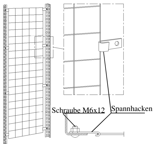
Drahtgitter-Seitenwand
