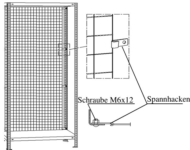
Drahtgitter-Rückwand
